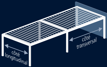
Couplage dans le sens de la largeur (adossées au mur, installations les unes derrière les autres) 24 mètres max.
