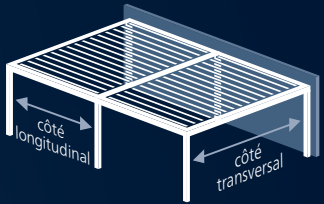
Couplage dans le sens de la longueur (installations côte à côte le long du mur) 18 mètres max.
