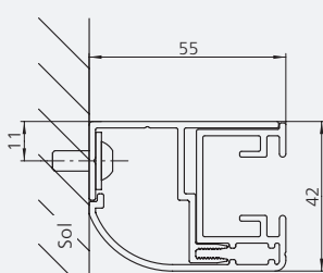
Montage intrados
