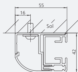
Montage mural
