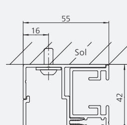
Montage mural
