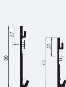
Consoles murales pour cassettes 75 et 92 mm
