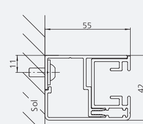
Montage intrados
