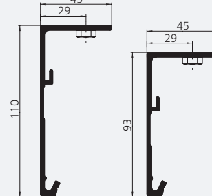
Consoles de plafond pour cassettes 75 et 92 mm
