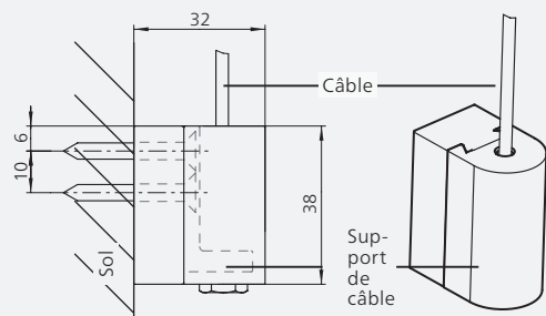
Montage au mur et intrados
