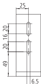
Équerre de fixation pour porte-cassette
