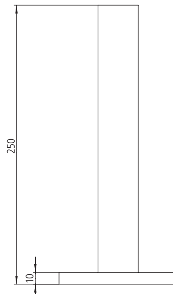
Socle pour le mât à visser
